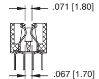
DETAIL A-A
