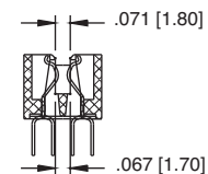
DETAIL A-A
