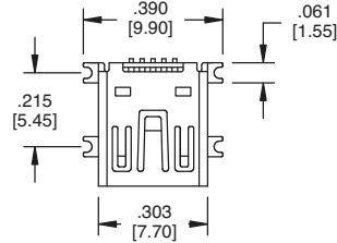
MUSB-AB1-S-RA-TSMT
