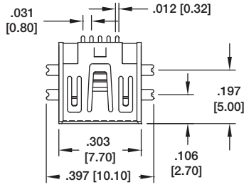
MUSB-AB-S-RA-TSMT
