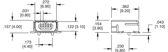
MUSB-AB1-S-RA-TSMT
