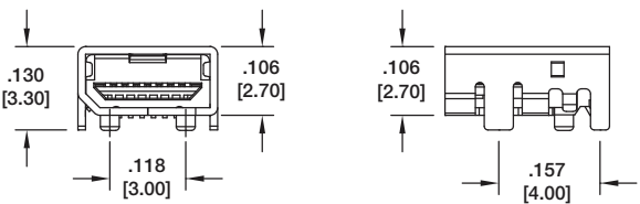
MUSB-8P-S-RA-SMT
