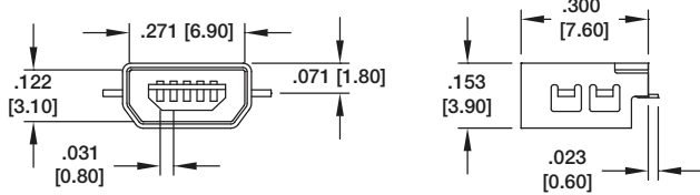
MUSB-AB-S-RA-TSMT
